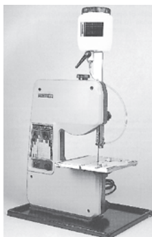
200234 Bandsäge „Proxxon“ Plangefräßer Arbeitstisch, um 45° schwenkbar. Geräuscharmer 230V Motor. Elektronisch regelbare Bandgeschwindigkeit von 120 - 250m/min Arbeitstisch 200 x 200mm. Inklusive Sägeblatt und Kühlmittelsystem
